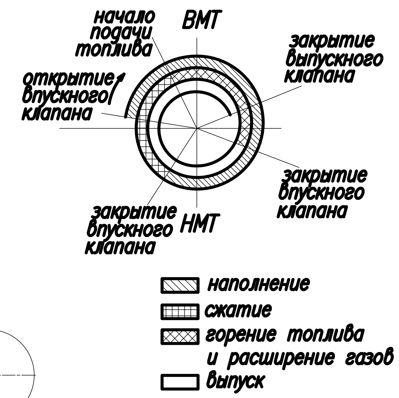
действительная диаграмма
