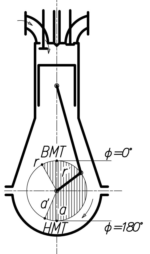
1-й такт
