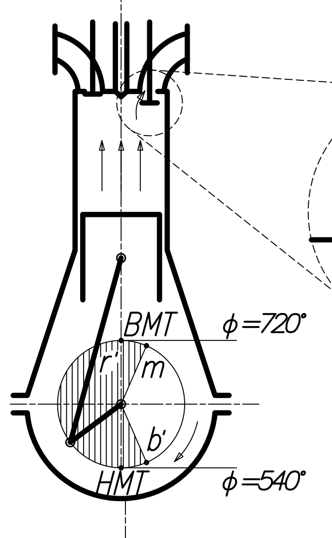
4-й такт
