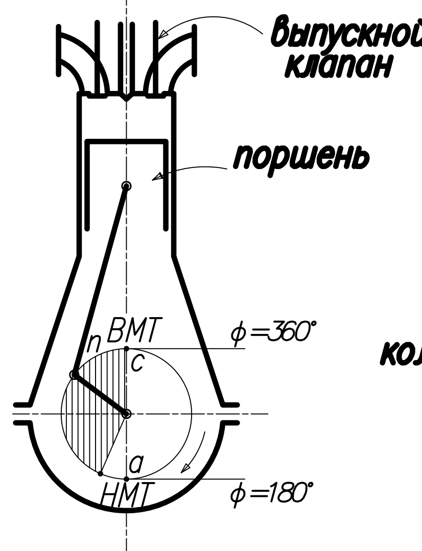
2-й такт
