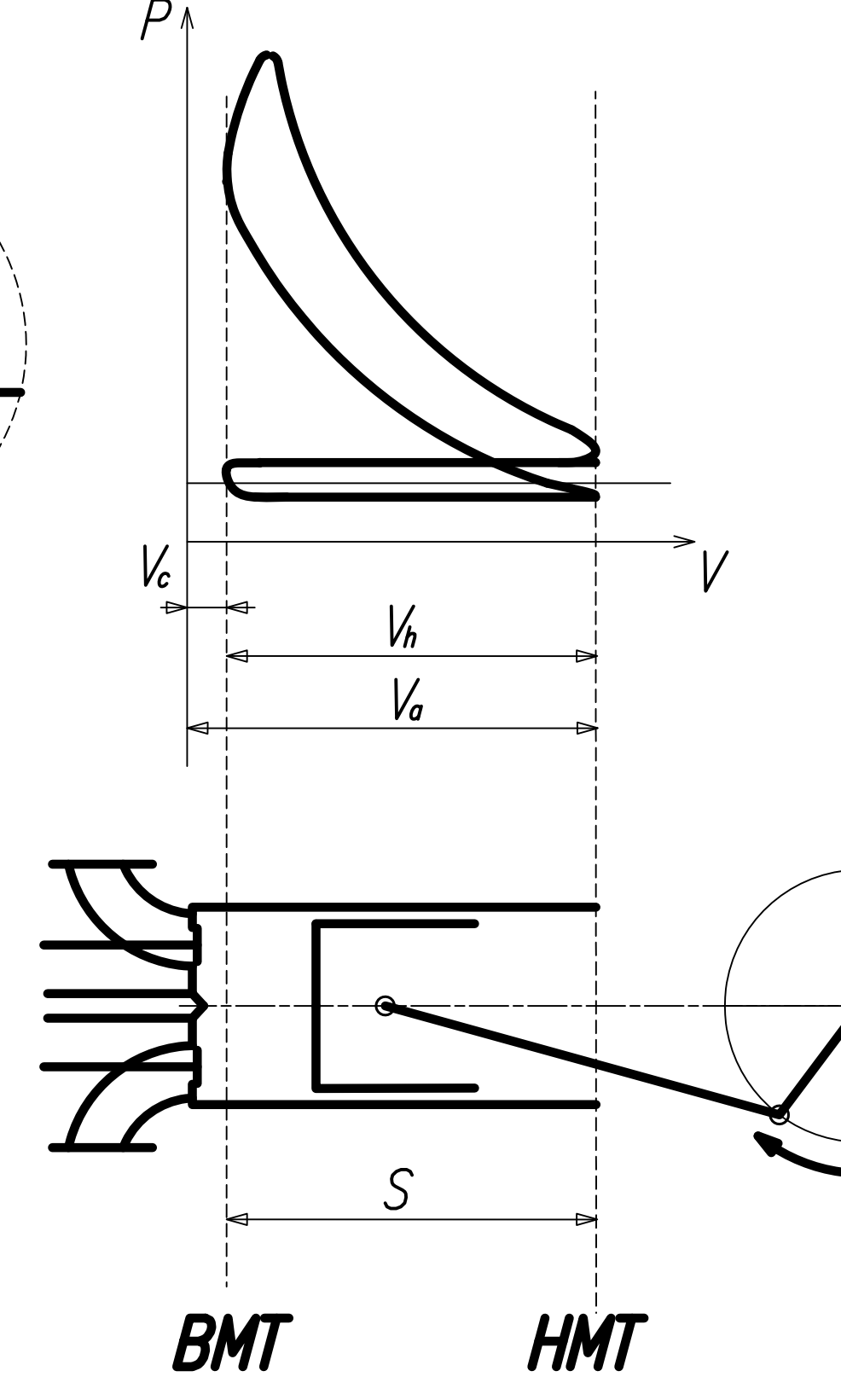
действительная диаграмма
