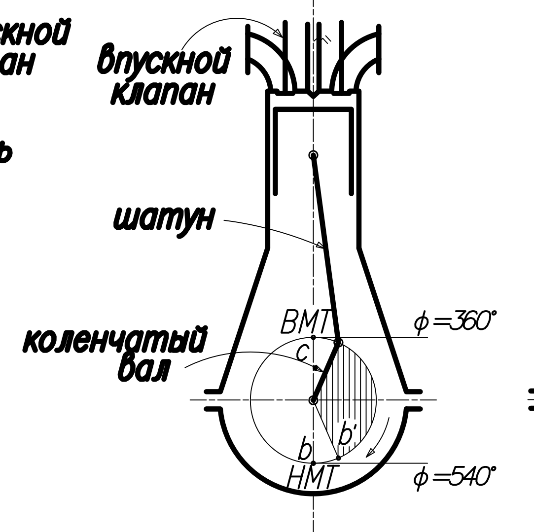
3-й такт
